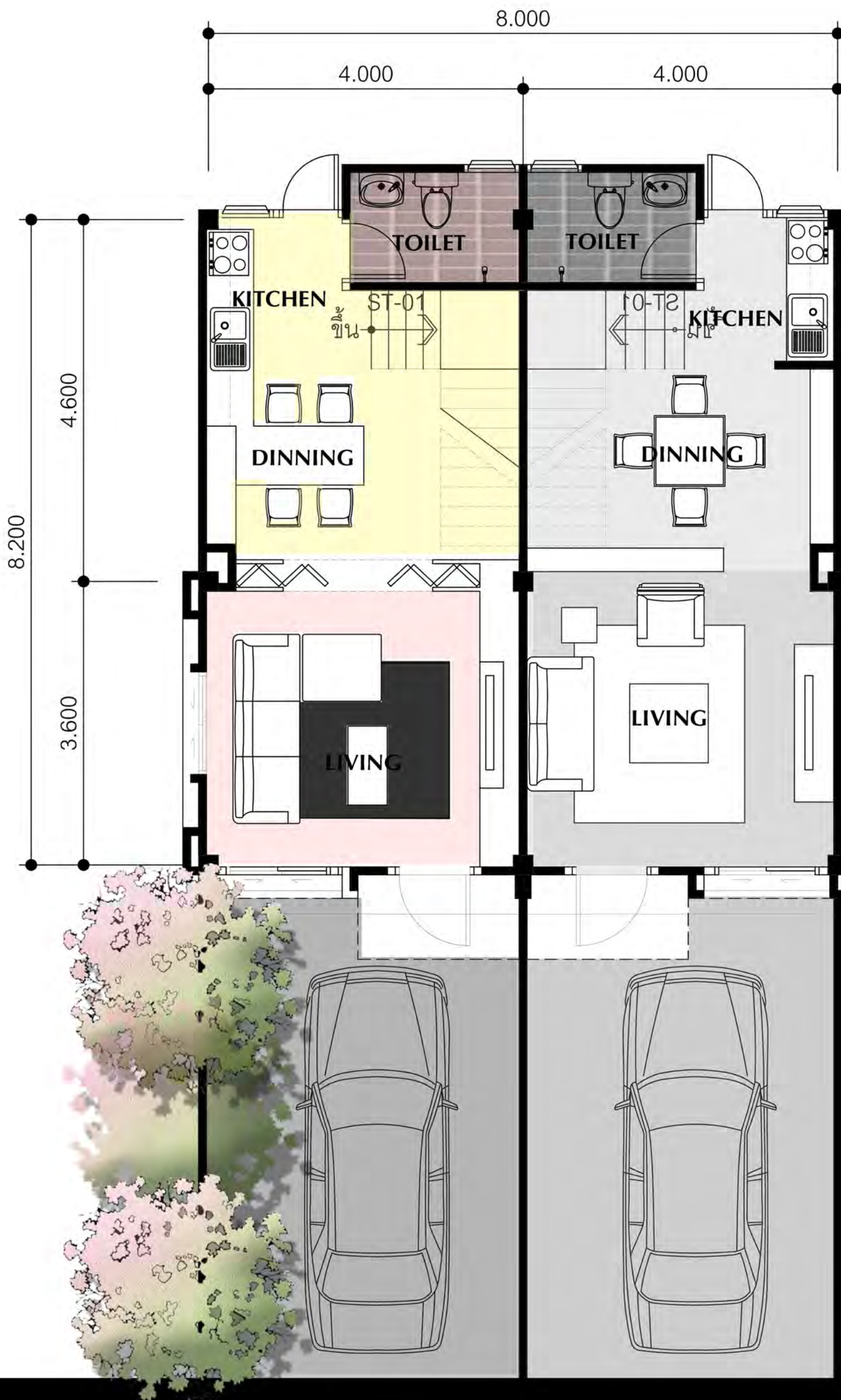
FLOOR PLAN 1 TOWN HOUSE : ทวีทรัพย์
